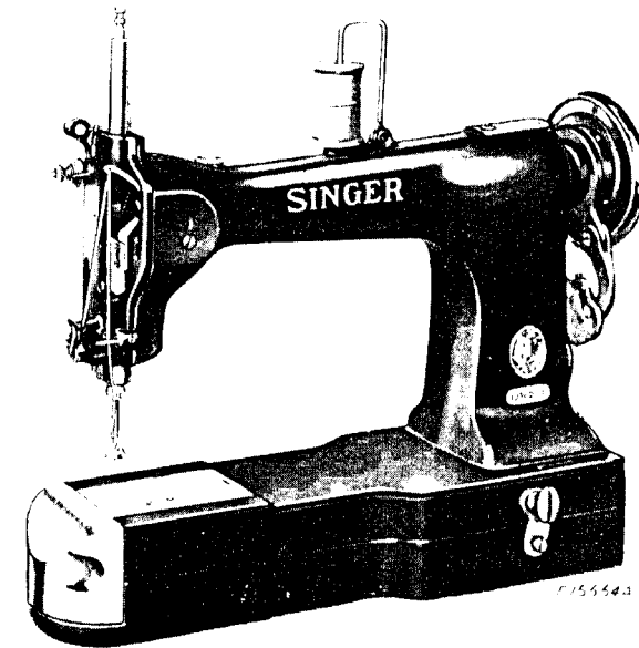
Fig. 1. Machine 12W223.
