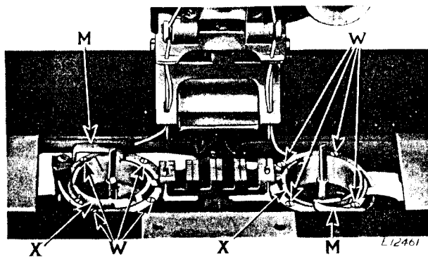
Fig. 20. Removing Bobbin Cases
